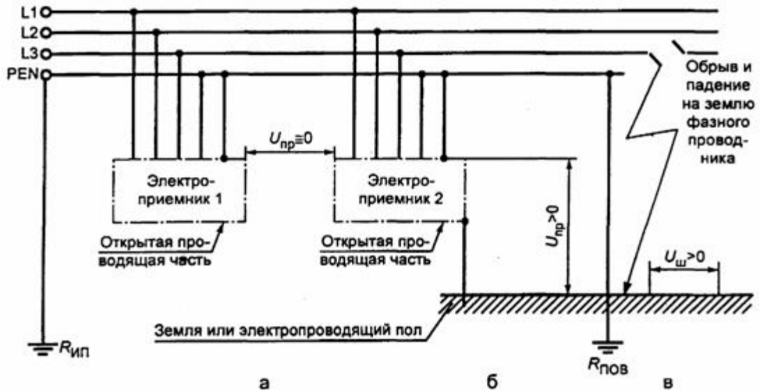
Рисунок В.4 — Сеть TN-C с замыканием на землю, например с оборванным и упавшим на землю фазным проводом U пр — напряжение прикосновения; U ш — шаговое напряжение; R ип — заземлитель источника питания; R пов — заземлитель для повторного заземления PEN-проводника В рассматриваемом аварийном режиме напряжения прикосновения на участке б) и шаговые напряжения на участках б) и в) могут длительно принимать значения, при которых возможно смертельное поражение электрическим током
