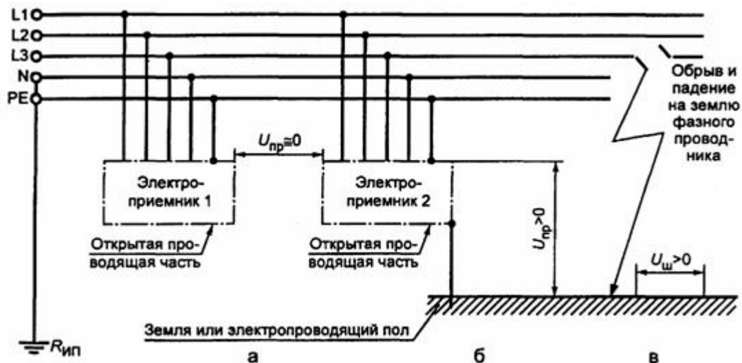
Рисунок В.5 — Сеть TN-S с замыканием на землю, например с оборванным и упавшим на землю фазным проводом U пр — напряжение прикосновения; U ш — шаговое напряжение; R ип — заземлитель источника питания В рассматриваемом аварийном режиме напряжения прикосновения на участке б) и шаговые напряжения могут длительно принимать значения, при которых возможно смертельное поражение электрическим током
