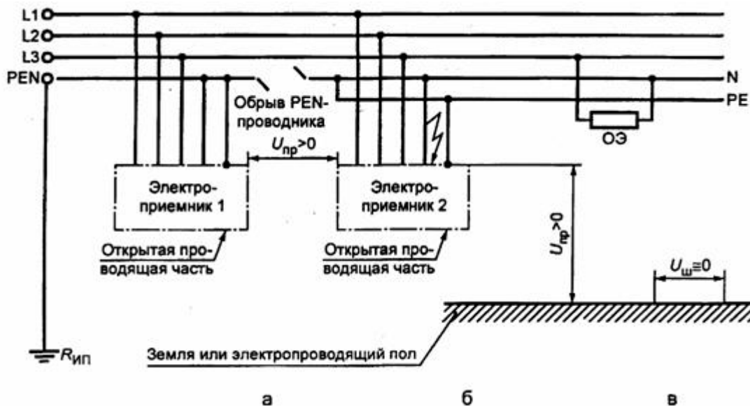
Рисунок В.7 — Сеть TN-C-S с обрывом PEN-проводника U_{пр} — напряжение прикосновения; U_{ш} — шаговое напряжение; R_{ип} — заземлитель источника питания; ОЭ — однофазный электроприемник В рассматриваемом аварийном режиме напряжения прикосновения на участках а), б) и шаговые напряжения на участке б) могут длительно принимать значения, при которых возможно смертельное поражение электрическим током
