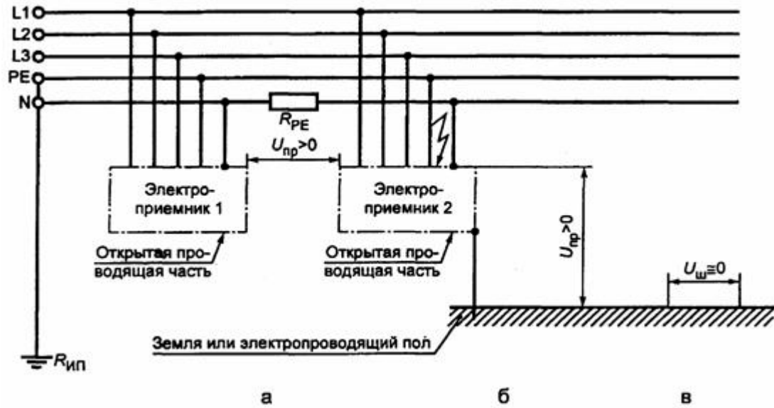
Рисунок В.6 — Сеть TN-S с однофазным замыканием на корпус U_{пр} — напряжение прикосновения; U_{ш} — шаговое напряжение; R_{ип} — заземлитель источника питания; R_{PE} — сопротивление PE-проводника В рассматриваемом аварийном режиме напряжения прикосновения на участках а), б) и шаговые напряжения на участке б) могут до момента срабатывания защиты принимать значения, при которых возможно смертельное поражение электрическим током
