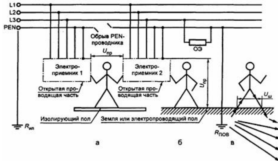
Рисунок В.1 — Сеть TN-C с оборванным PEN-проводником.
