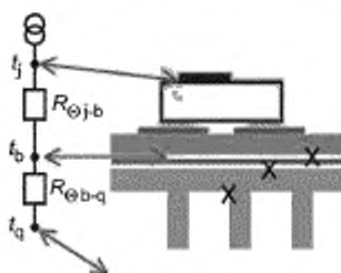
Рисунок 1 — Схематическое изображение цепочки тепловых сопротивлений светильника с СД
