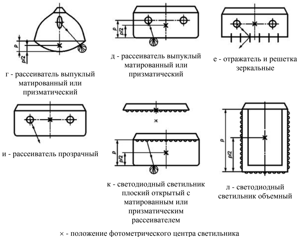
Рисунок В.1 - Положение фотометрического центра осветительного прибора
