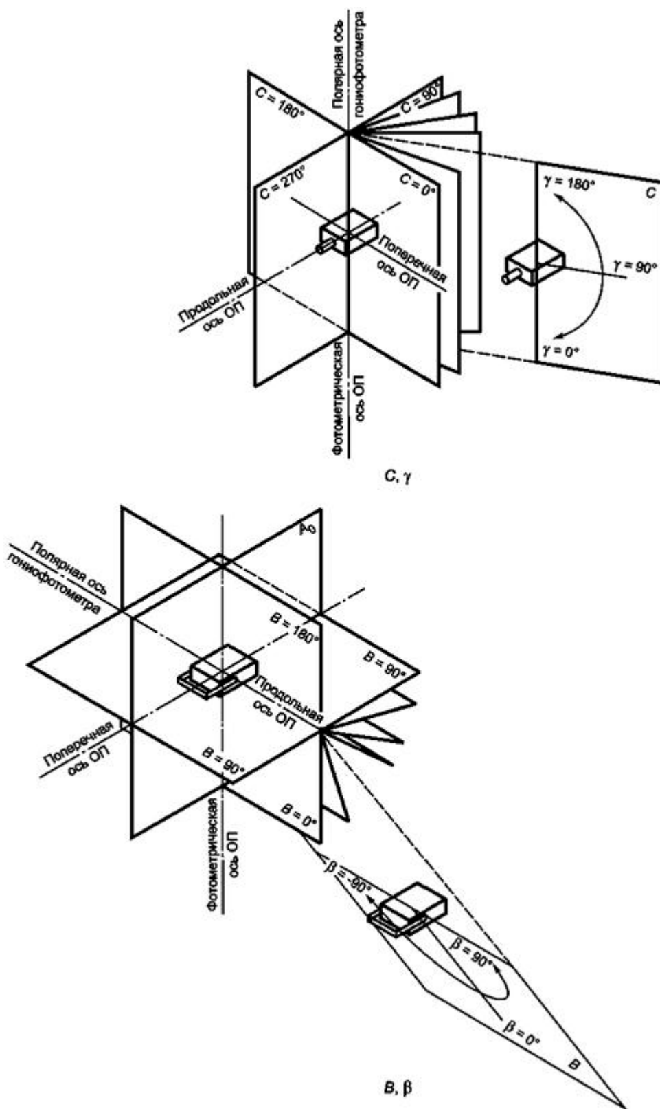
Рисунок Б.1 - Системы фотометрирования, лист 1
